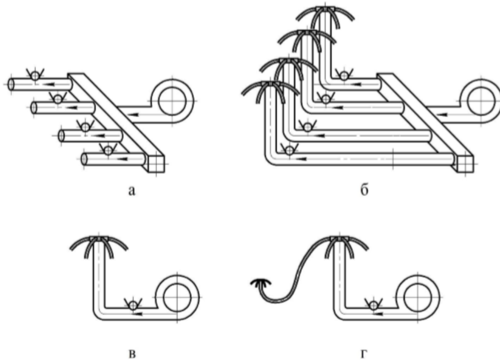
Рис. 2. Схеми розподільних систем пневматичних зернових сівалок: а – безступінчаста індивідуального дозування; б – двоступенева групового дозування; в – одноступенева загального дозування; г – двоступенева загального дозування.
